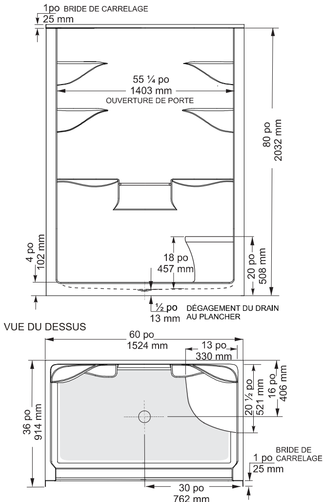
D'ÉVACUATION CENTRE - DOUCHE GAUCHE ILLUSTRÉ VUE DE DEVANT
